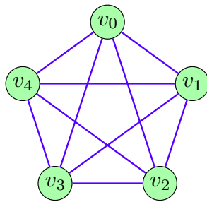
K_5
