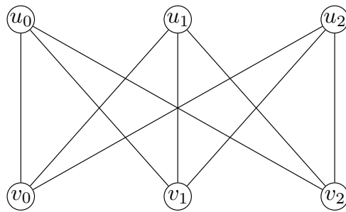
K_{3,3}
